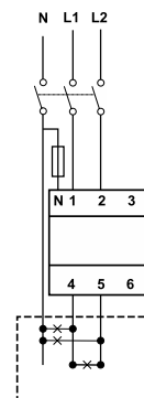
图7双相系统(3线)
